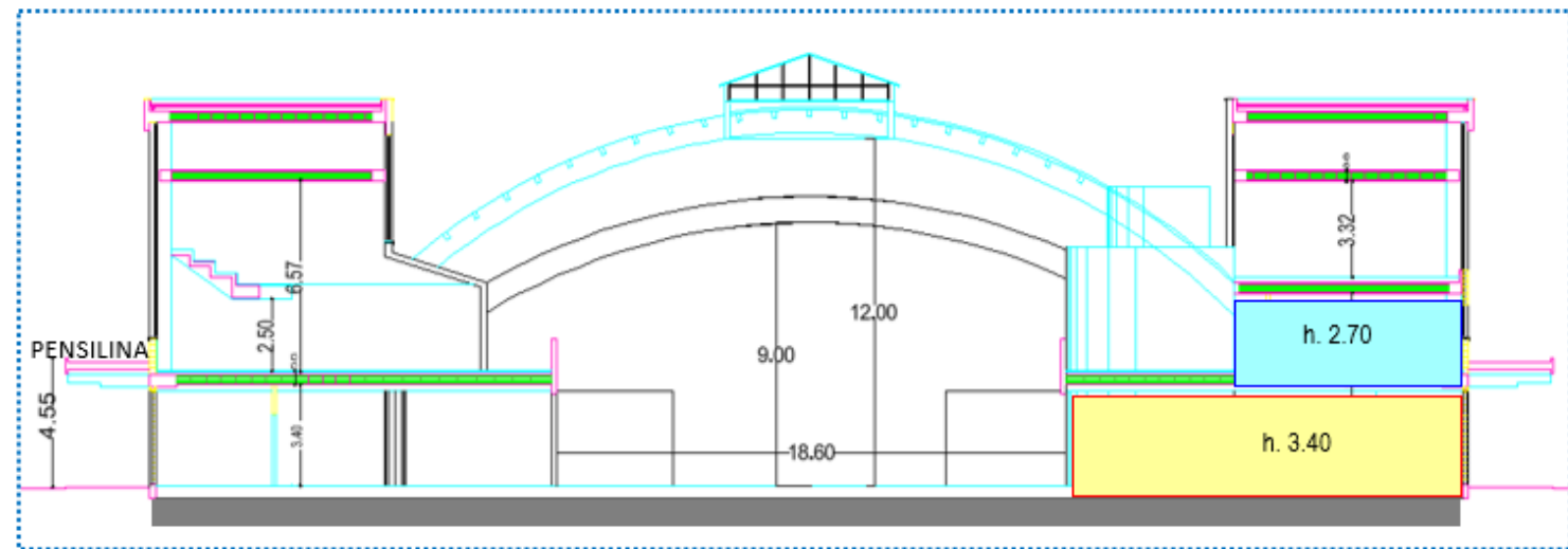
SEZIONE
